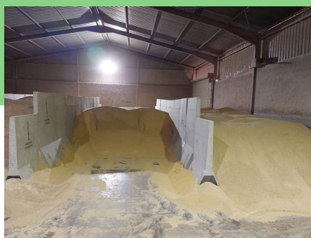
Met ReMaCon se Yfel-paneel kan 'n boer sy skuur inrig soos dit hom pas en verander as behoeftes verander. By Butt Farming is dit noodsaaklik dat die trok vir aflaai en die laai-graaf wat die materiaal weer moet kom oplaai maklik toegang het.
